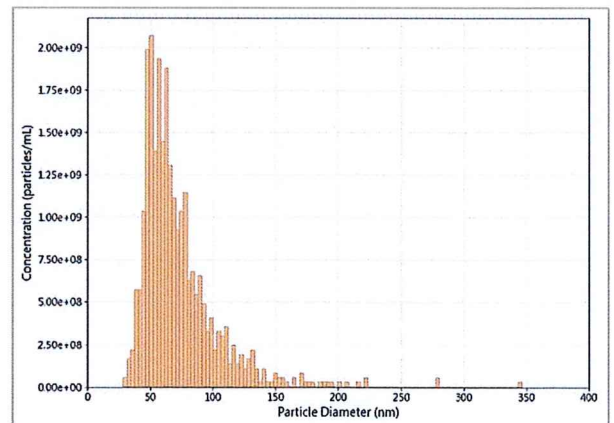
粒徑分布圖：
