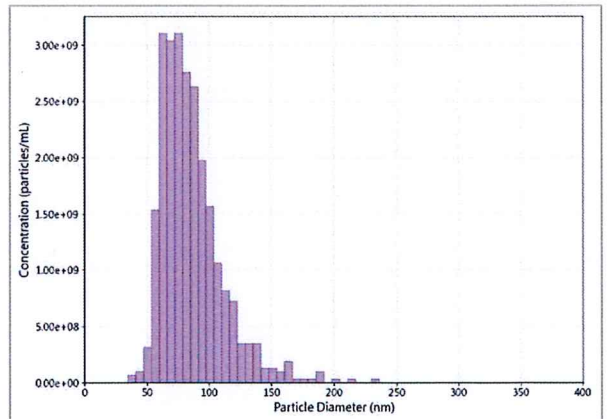
粒徑分布圖：
